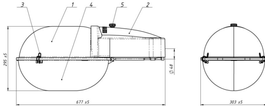
Рисунок 1. Светильник РКУ16
