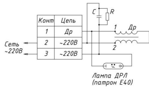
Схема электрическая светильников РКУ16 (Лампа ДРЛ в комплект поставки светильника не входит)
